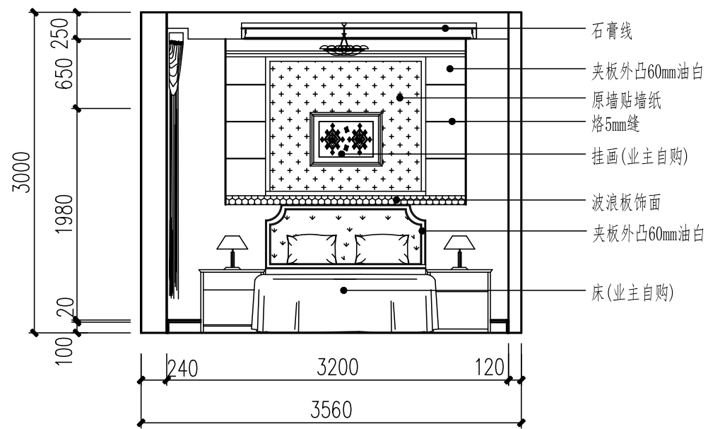
次卧背景B立面图 1:50
