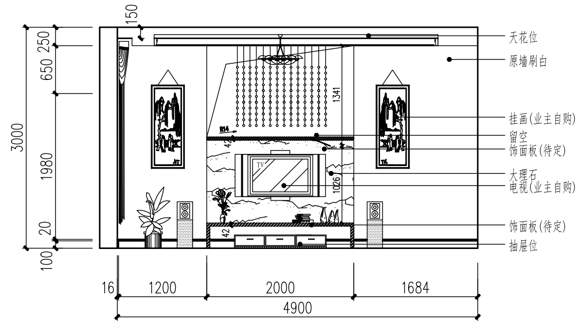
客厅背景A立面图 1:50
