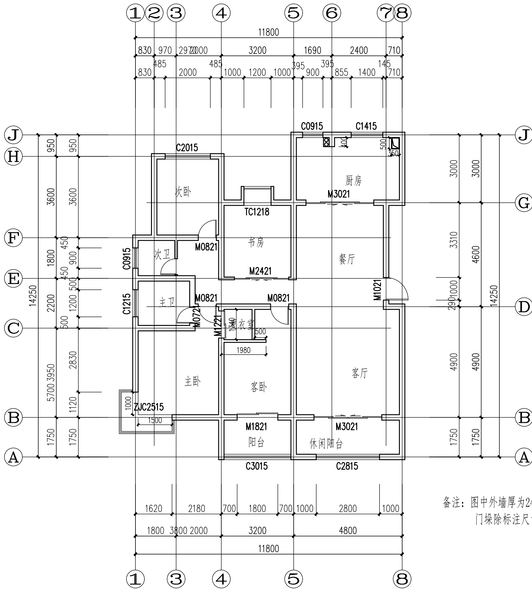
建筑平面图 1:100
