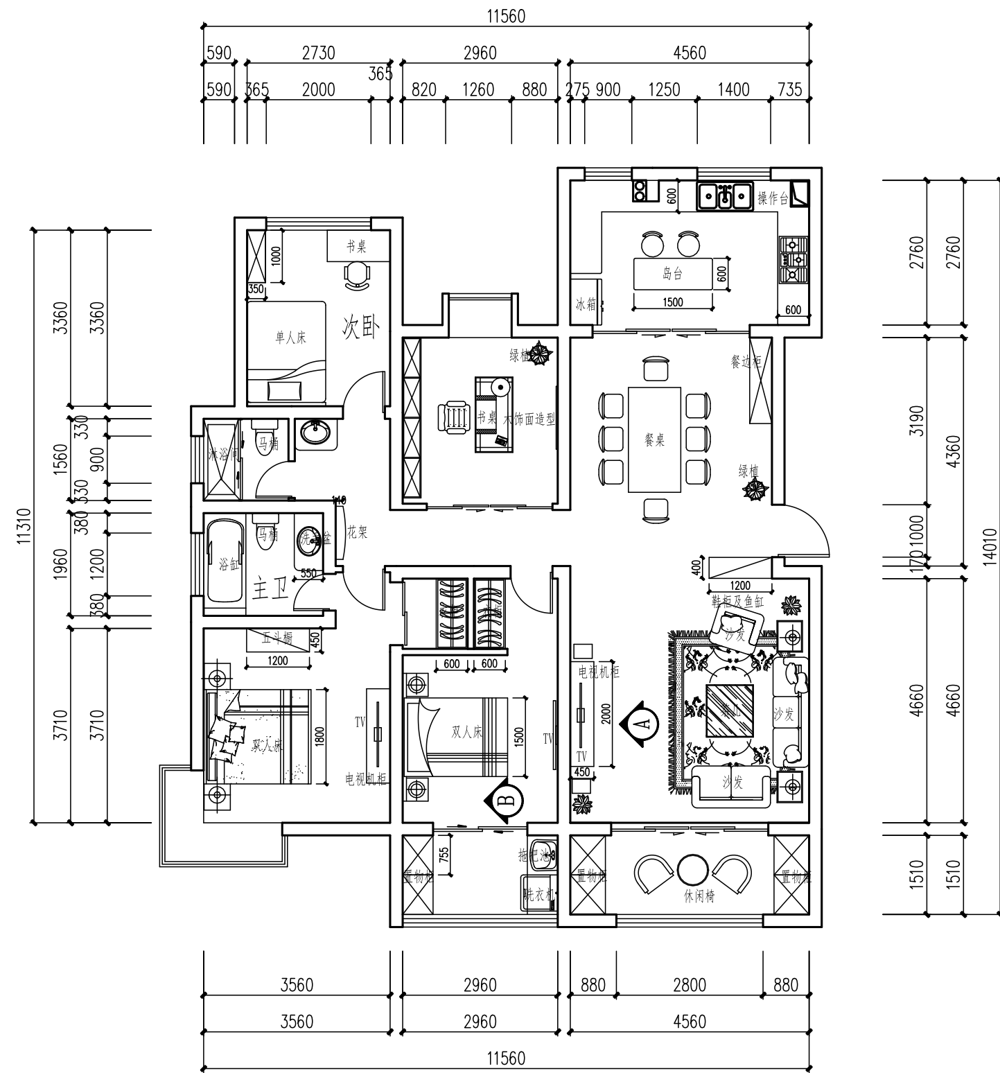
家具平面布置图 1:100
