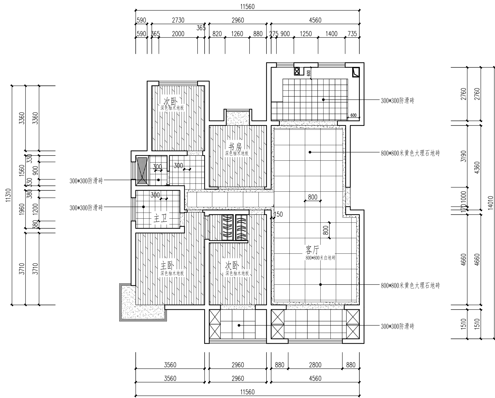
地面布置图 1:100
