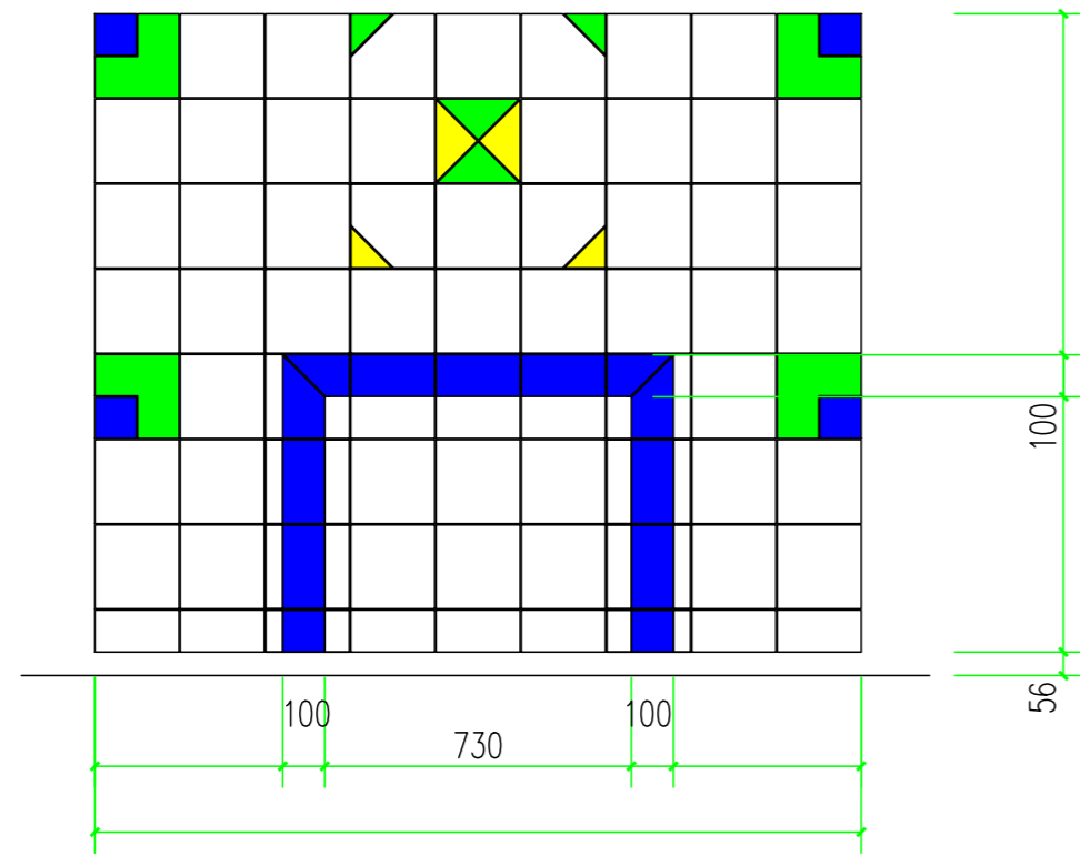
墙面拼花组合示意图
